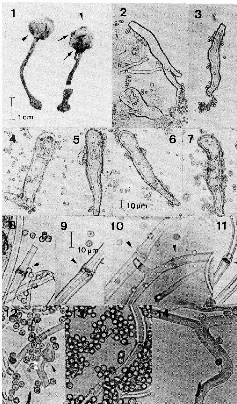
Figs. 1-14. Tulostoma cyclophorum Lloyd, (H.AH 11615), 1, cuerpos fructíferos; 2-7, "mycosclereids"; 8-14, septos del capillicio.
