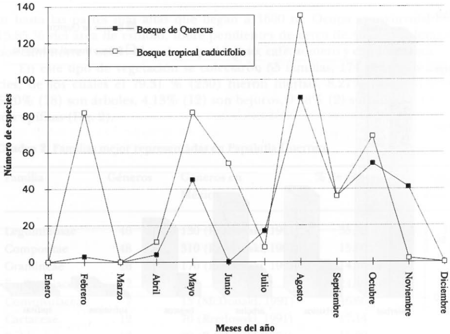
Fig. 3. Floración y/o fructificación por tipo de vegetación.
