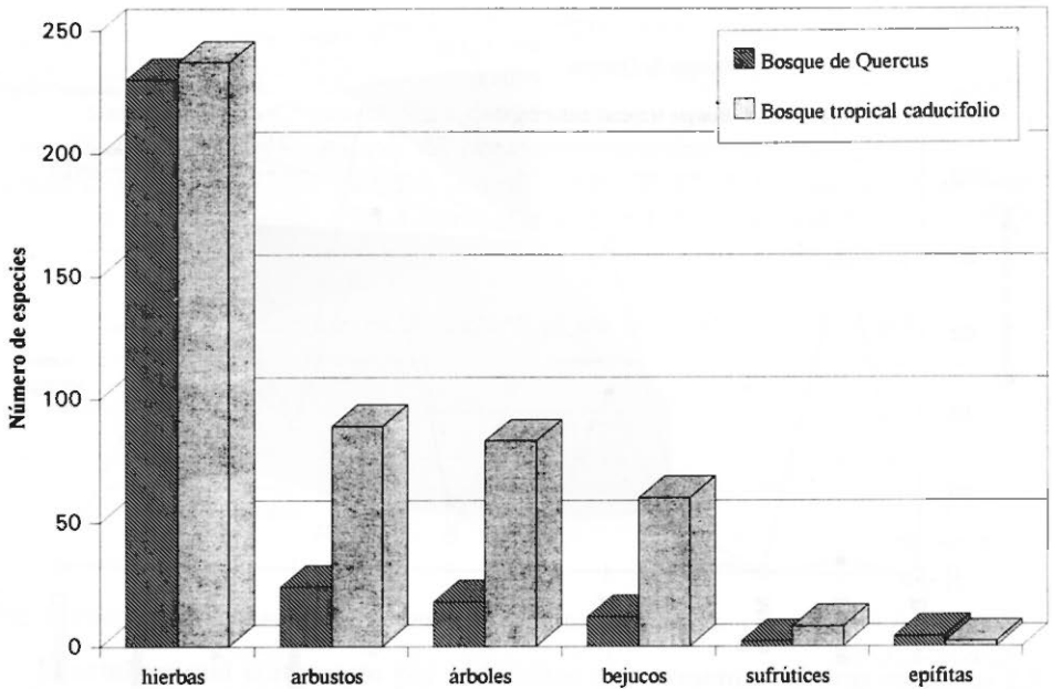
Fig. 2. Formas de vida por tipo de vegetación..
