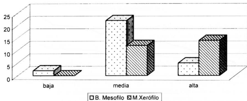
Fig. 1. Distribución de la gravedad específica de las especies de bosque mesófilo y matorral xerófilo. Las especies del matorral xerófilo muestran gravedad específica más alta.
